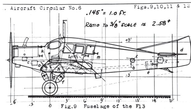
Ўрта Осиё фуқаролик авиацияси учун харид қилинган «Junkers F-13» аэропланининг чизмаси
